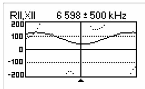
wykres R||,X|| - model równoległy
