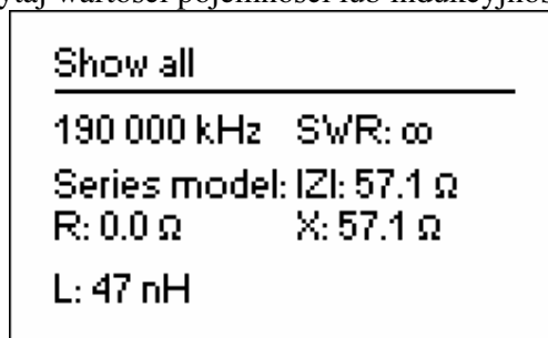
Przykład 2: Nieznana indukcyjność
