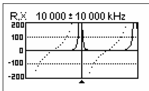
kabel rozwarty
